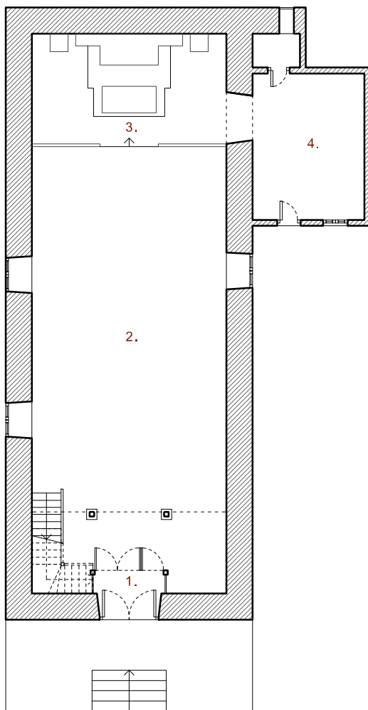
PLANTA PRIMER NIVEL
