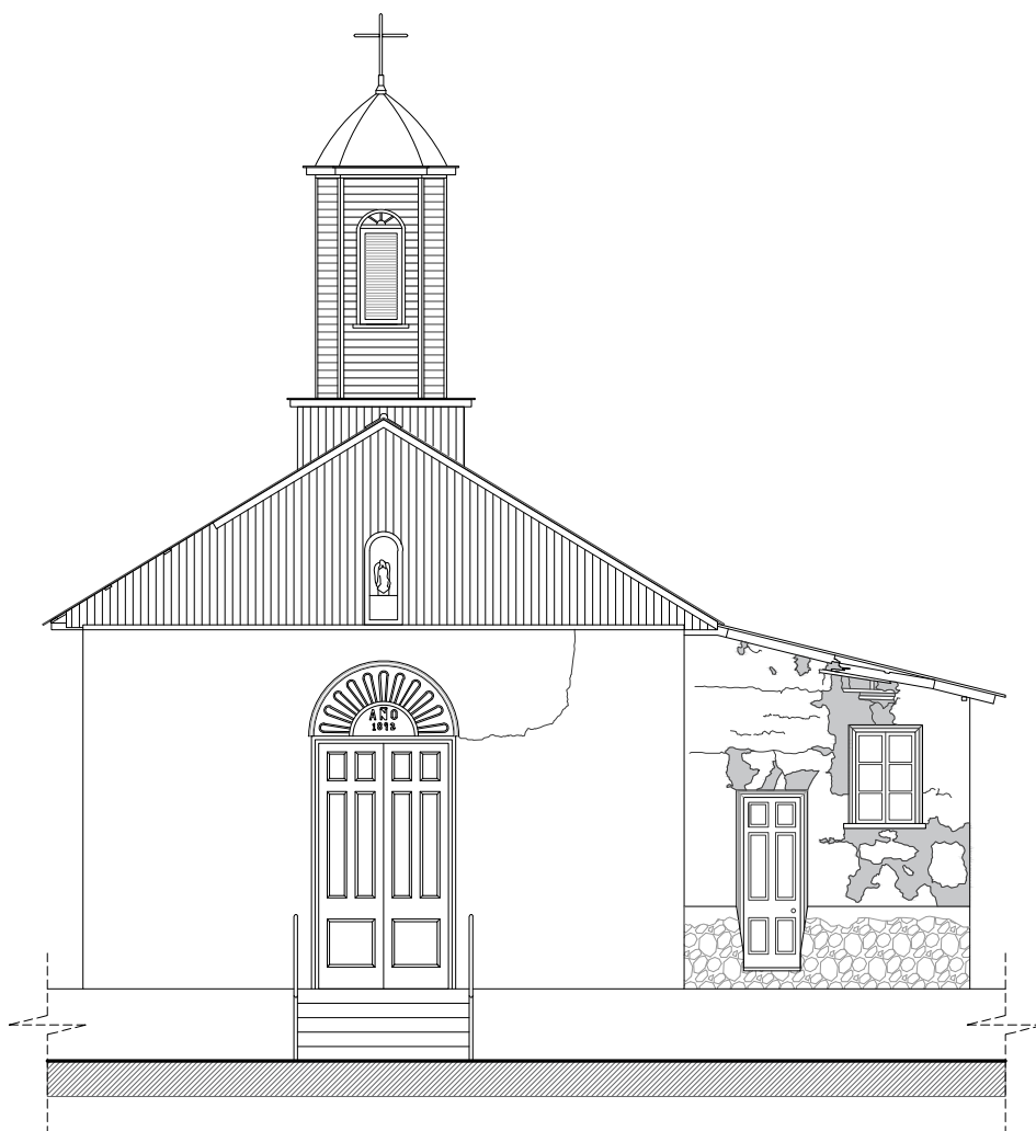
ELEVACIÓN FACHADA
