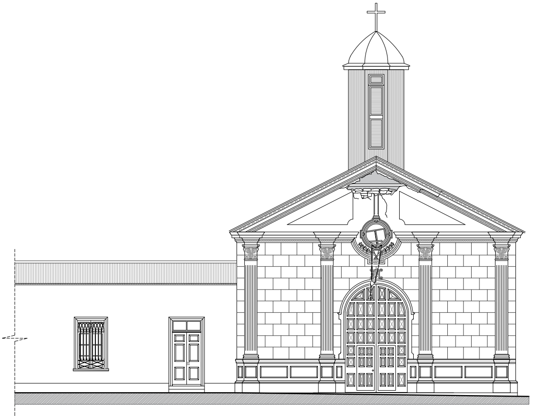
ELEVACIÓN FACHADA
